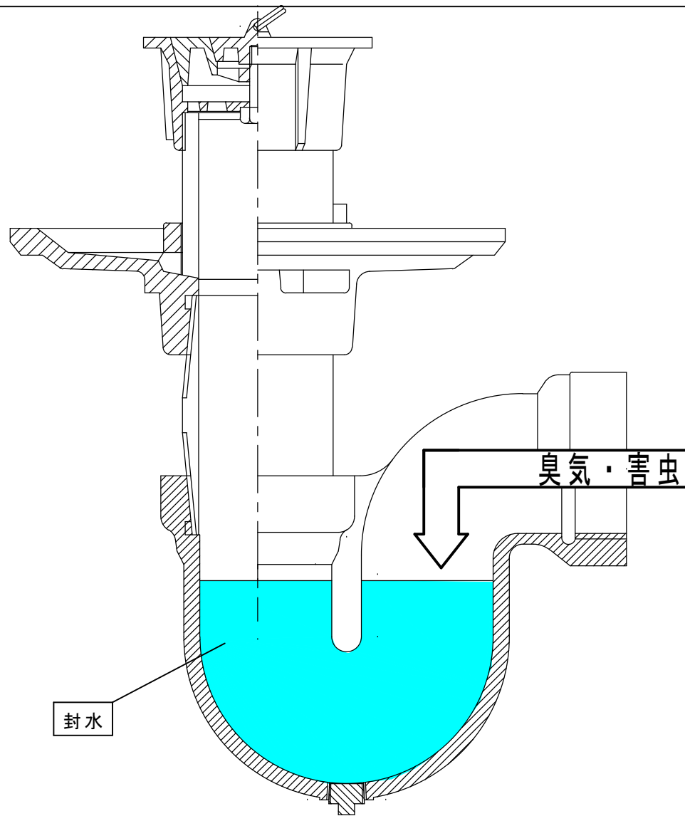
P型トラップ（手洗い等）
