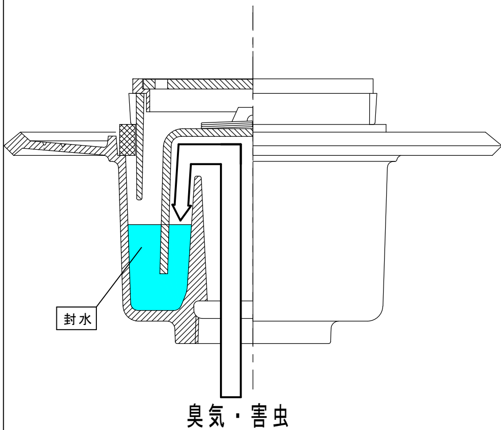
椀型トラップ（床掃除口等）
